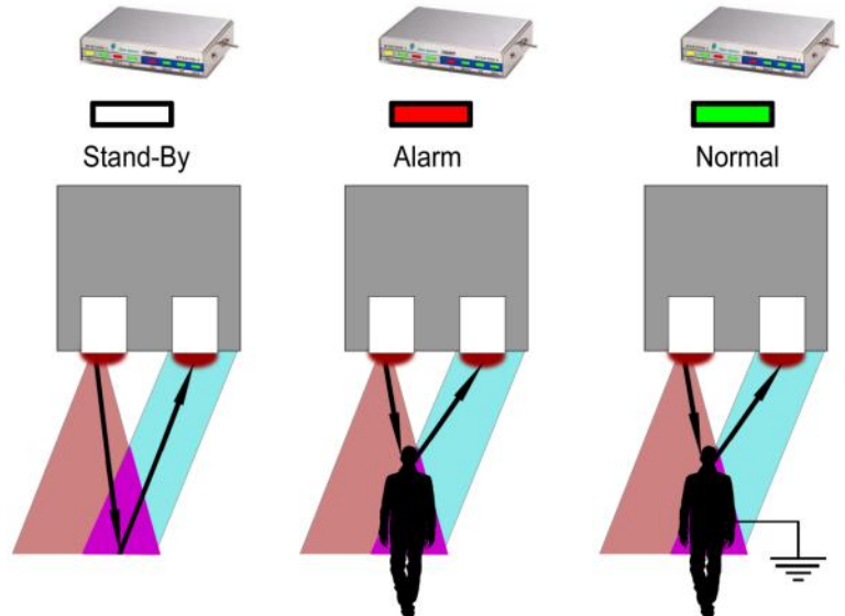
CM-Remote IR Alarm Examples
